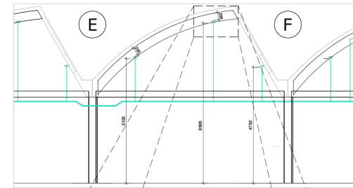
Schnitt A-A (Achse E-F / 9-11) M 1:50 0 0.5 1.0 2.0
